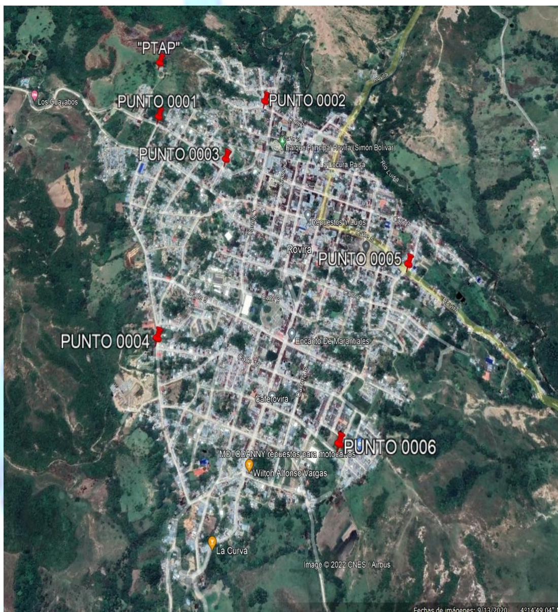
IMAGEN SATELITAL DE PUNTOS DE MONITOREO ACUEDUCTO URBANO DEL MUNICIPIO DE ROVIRA
