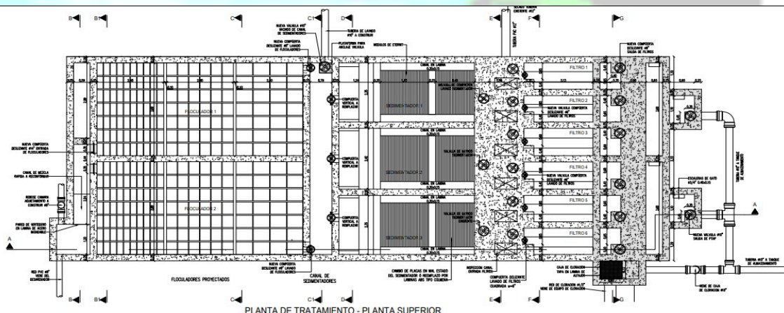
Levantamiento estructura Planta de Tratamiento
