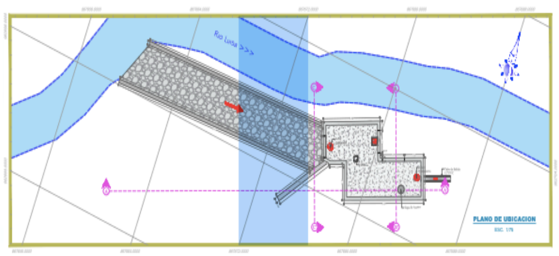
Levantamiento Estructura Bocatoma
